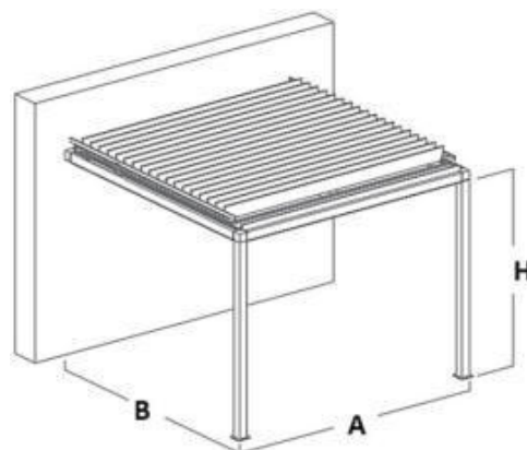
Fassaden Montage
