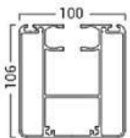
Führungprofil
